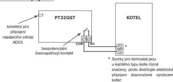
Schéma zapojení:
